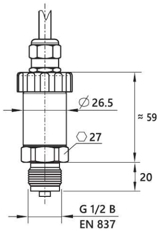
Cable Outlet
